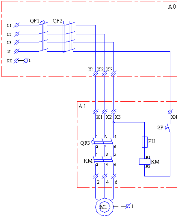
Электрическая схема 1
